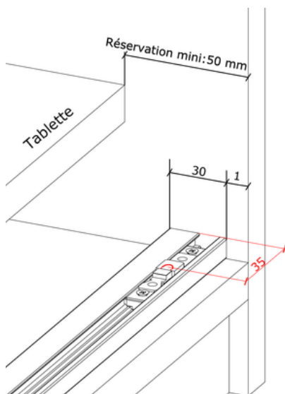
Vue perspective
