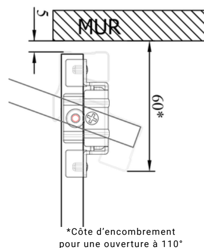
Vue dessus
