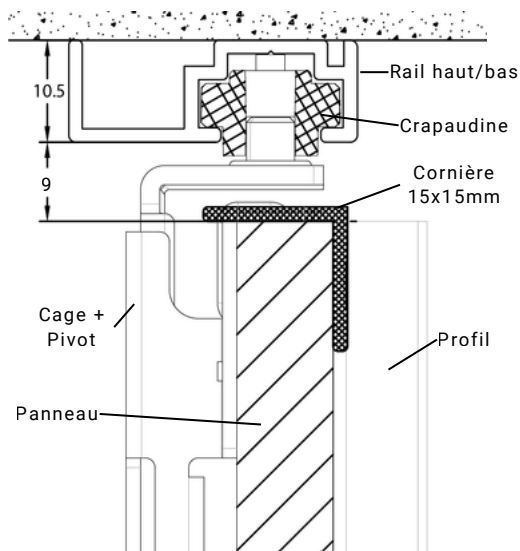
Vue en coupe
