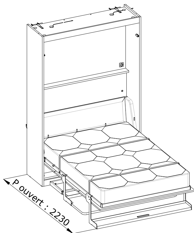
Version ouverte
