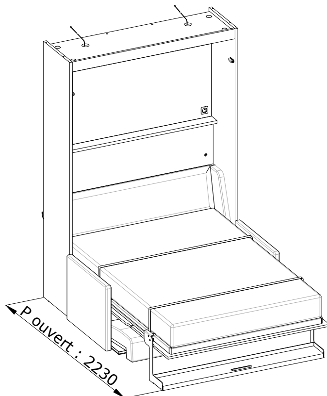
Version ouverte
