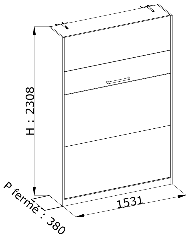
Version fermée
