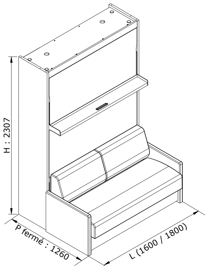
Version fermée
