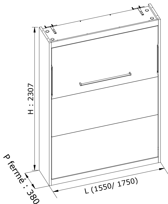
Version fermée
