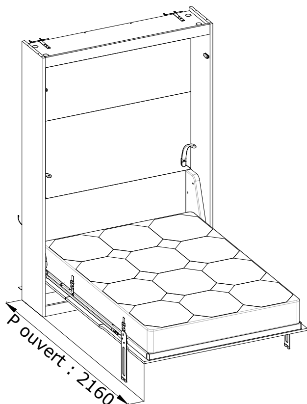
Version ouverte
